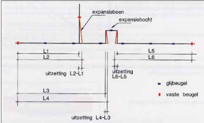
Figuur 4: Voorbeeld van expansiebocht bij vrijliggende leidingen.
